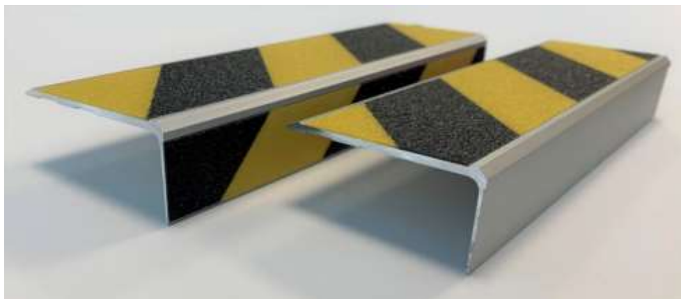
Beispiel: Treppenkanten 30 x 60 mm mit Einlage 50 mm gelb-schwarz beklebt, ohne und mit Setzstufenbeklebung mit 23 mm Einlage
